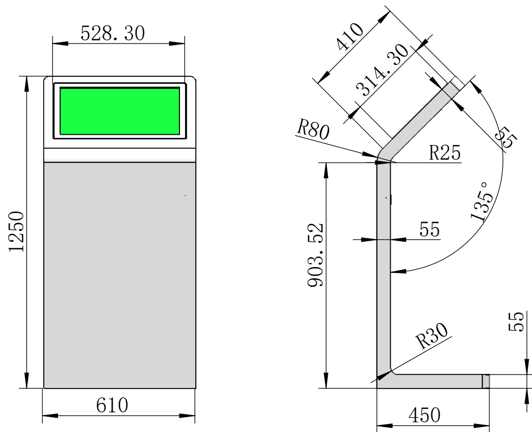
21.5寸L型斜面一体机外观尺寸图
